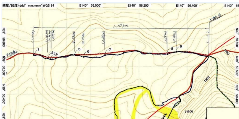
水切り設置位置図
